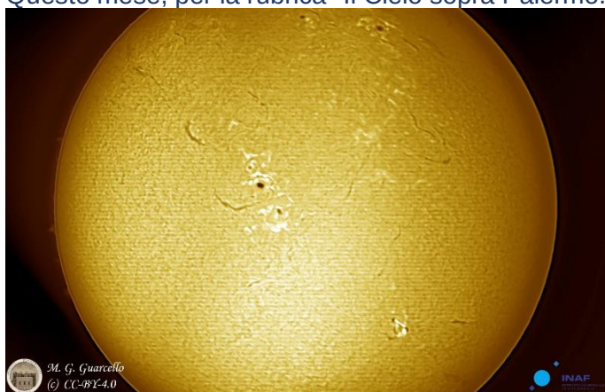
7 Febbraio: il Sole in Halpha
