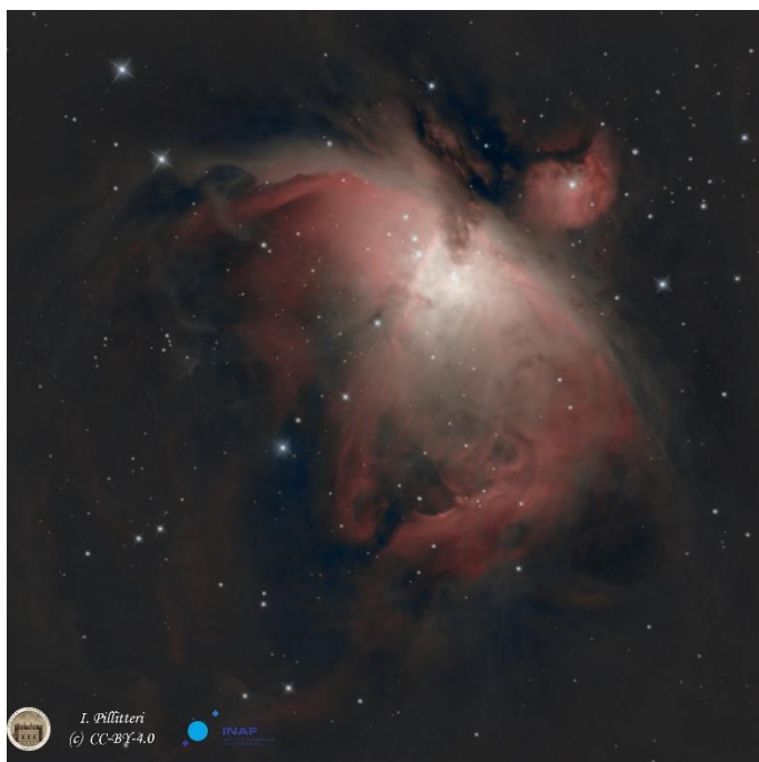
14 Febbraio: Nebulosa di Orione
