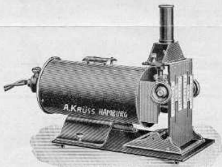
Mikro-Nephelometer Nr. 7015a (Liste Nr. 41) R.M. 395.—
